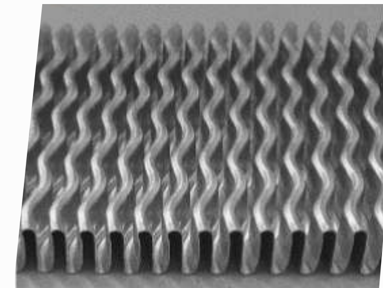
Wavy Fin
